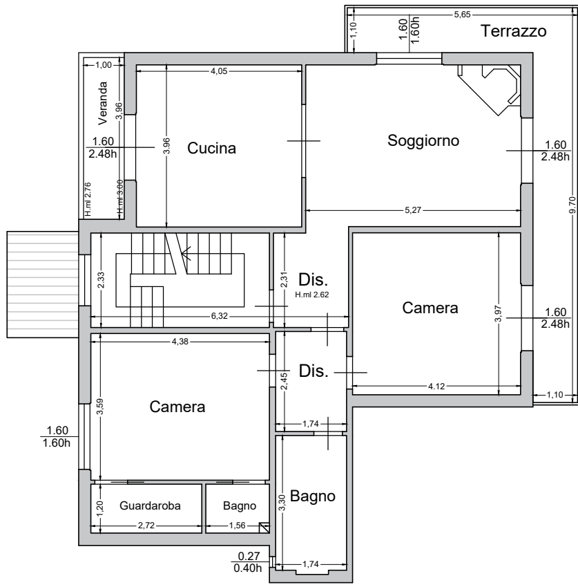
Piano Primo H.ml 2.95
