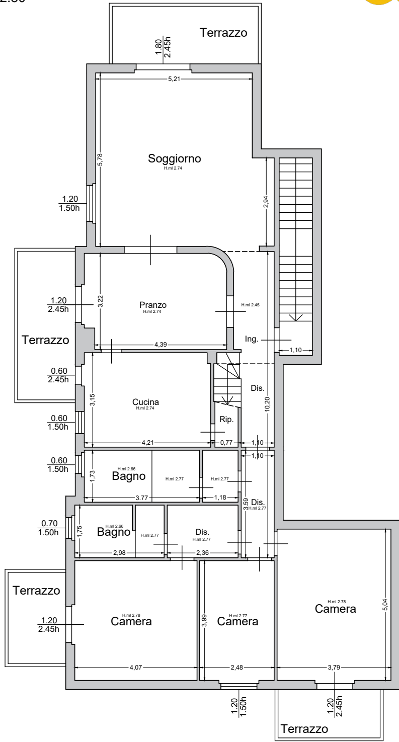
Piano Primo H.ml 2.80
