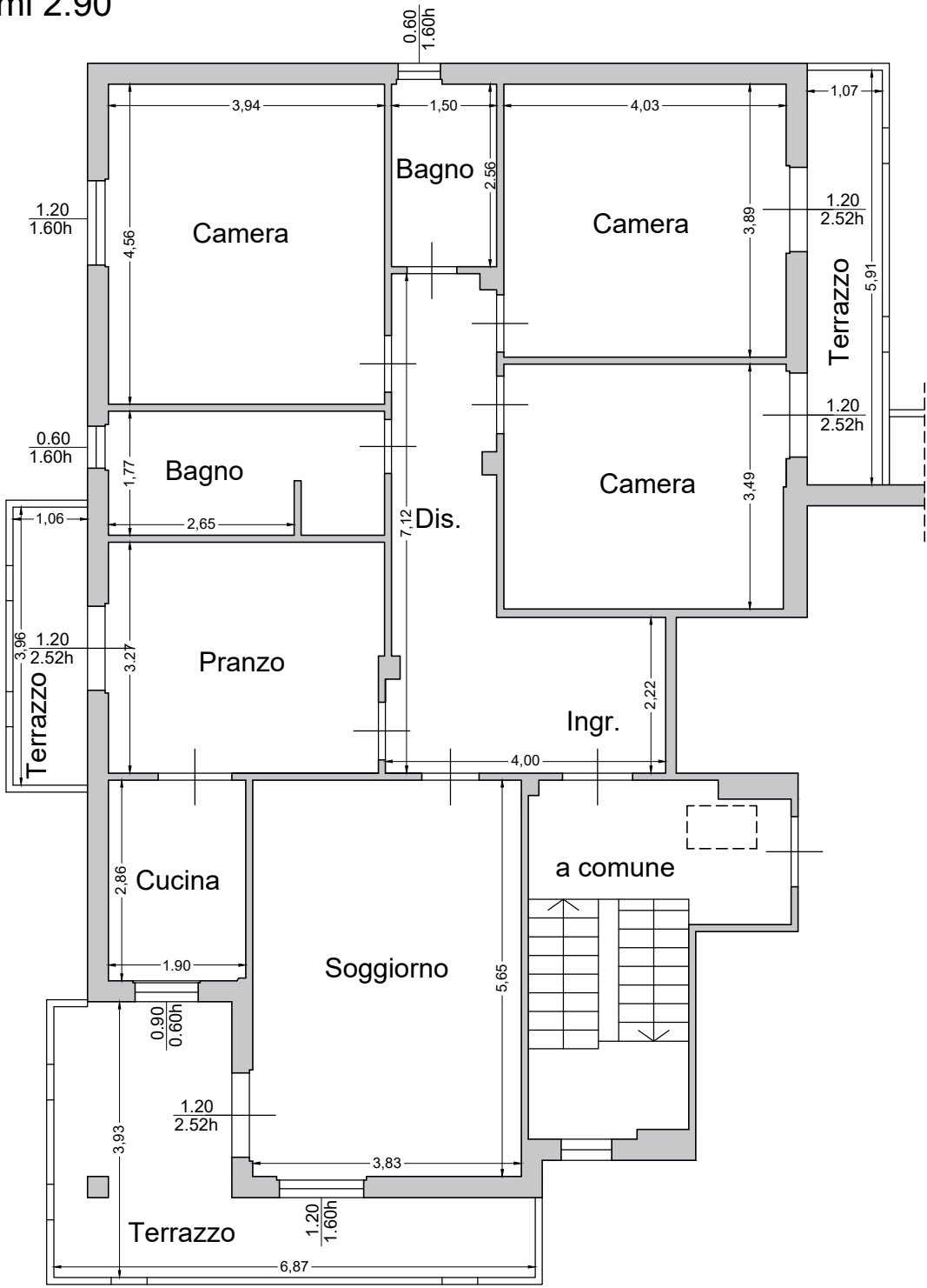
Piano Secondo H.ml 2.90
