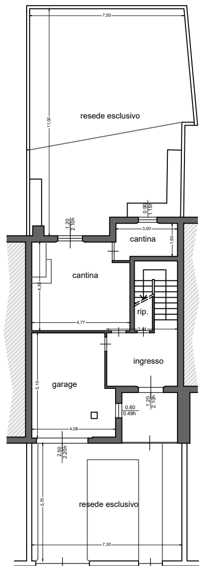
Pianta Piano PRIMO h 2,40 m
